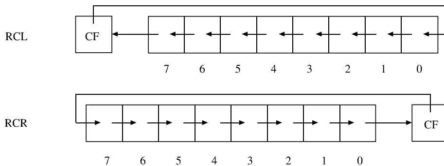
איור 5.26 הזזה מעגלית עם נשא
