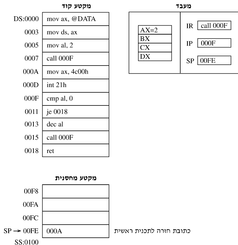
איור 7.14 מצב הזיכרון והמעבד לאחר קריאה לפונקציה example
