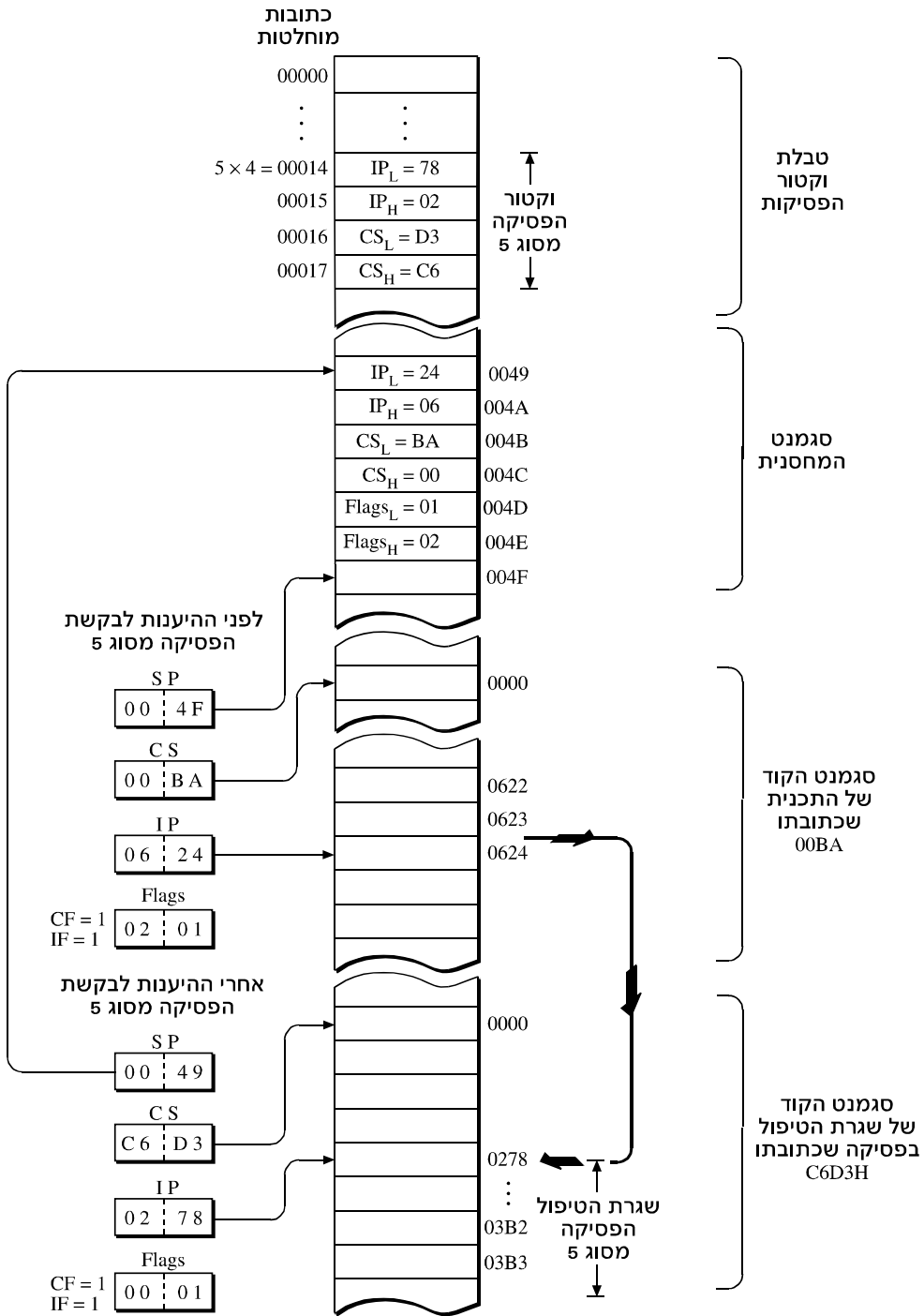
9.3 איור היענות לבקשת פסיקה מסוג 5
