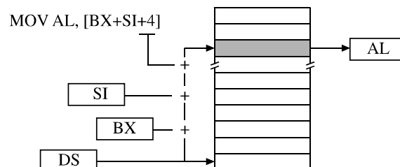
איור 6.8 מיעון אינדקס-בסיס עם העתק
