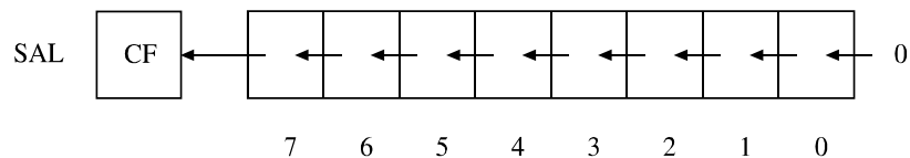
איור 5.22 הזזה אריתמטית שמאלה של בית
