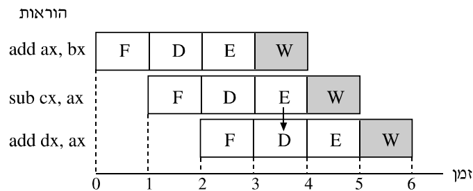
איור 10.12 שימוש בקידום נתונים
